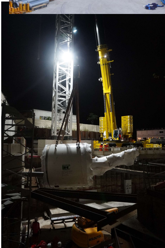
Photo du 26/06/2024 Descente d'un élément du tunnelier de nuit
